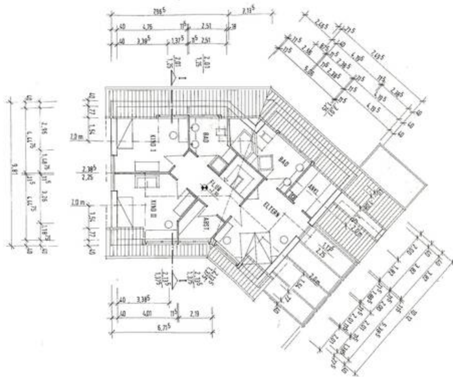
Grundriss OG
