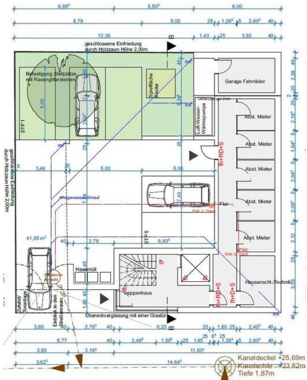
Grundriss Erdgeschoss
