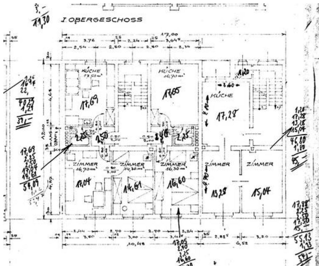
Grundriss 1.OG
