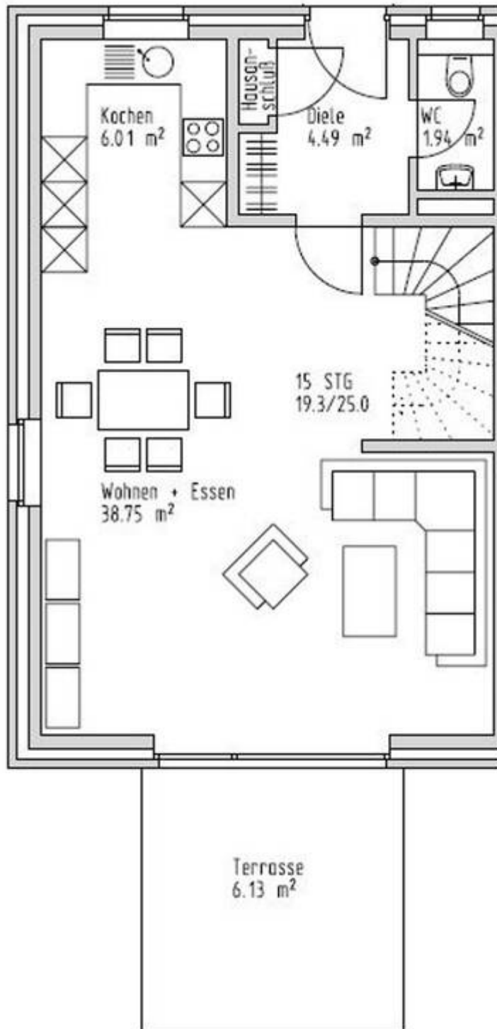
Grundriss Erdgeschoss
